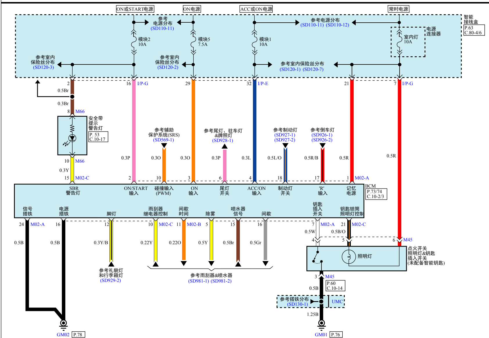
车身控制模块(BCM)系统(1)
